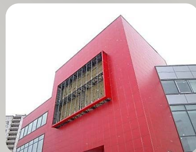
Металлоконструкция для светодиодного экран на фасаде торгового центра в г. Химки
